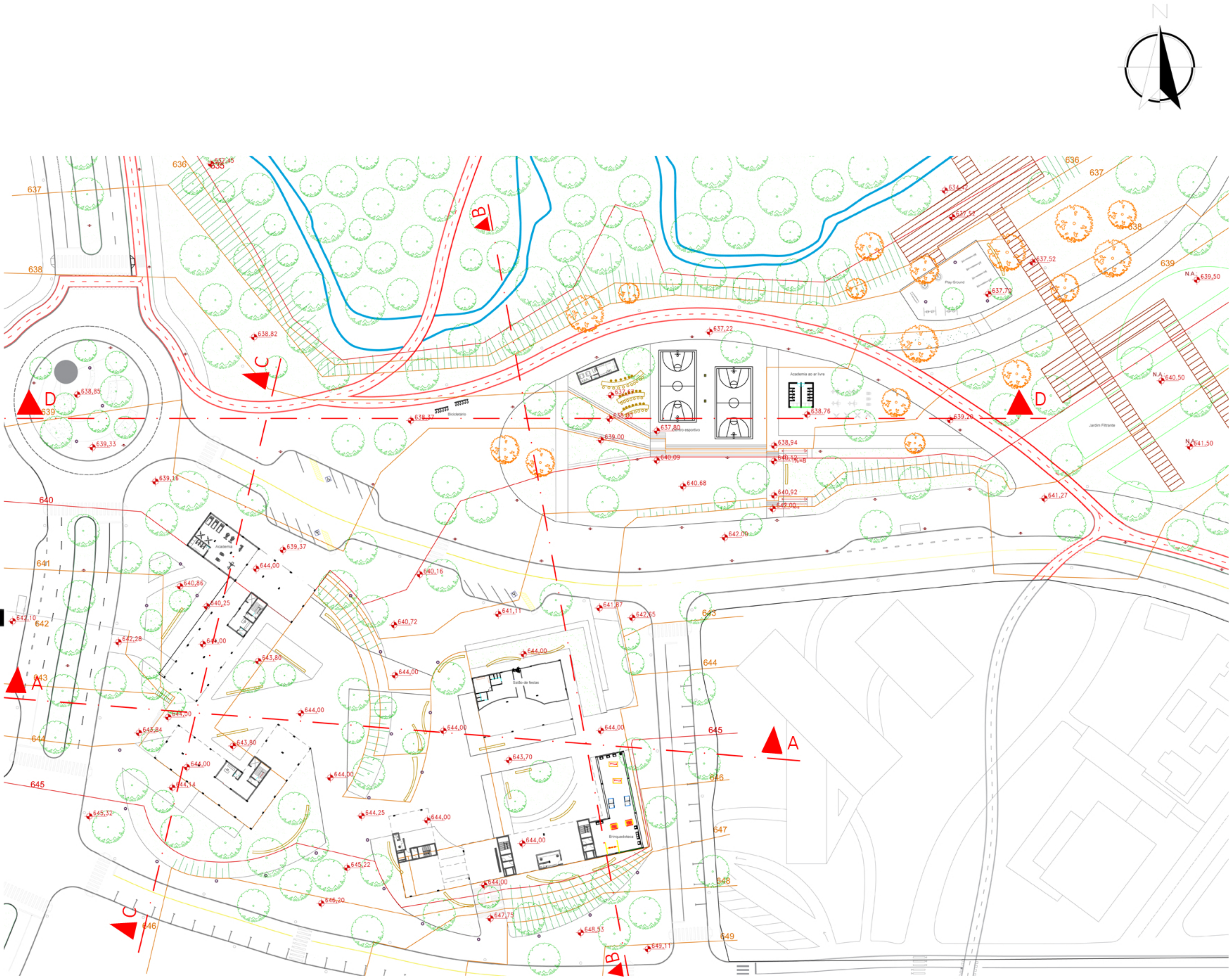
Implantação esc: 1:500
