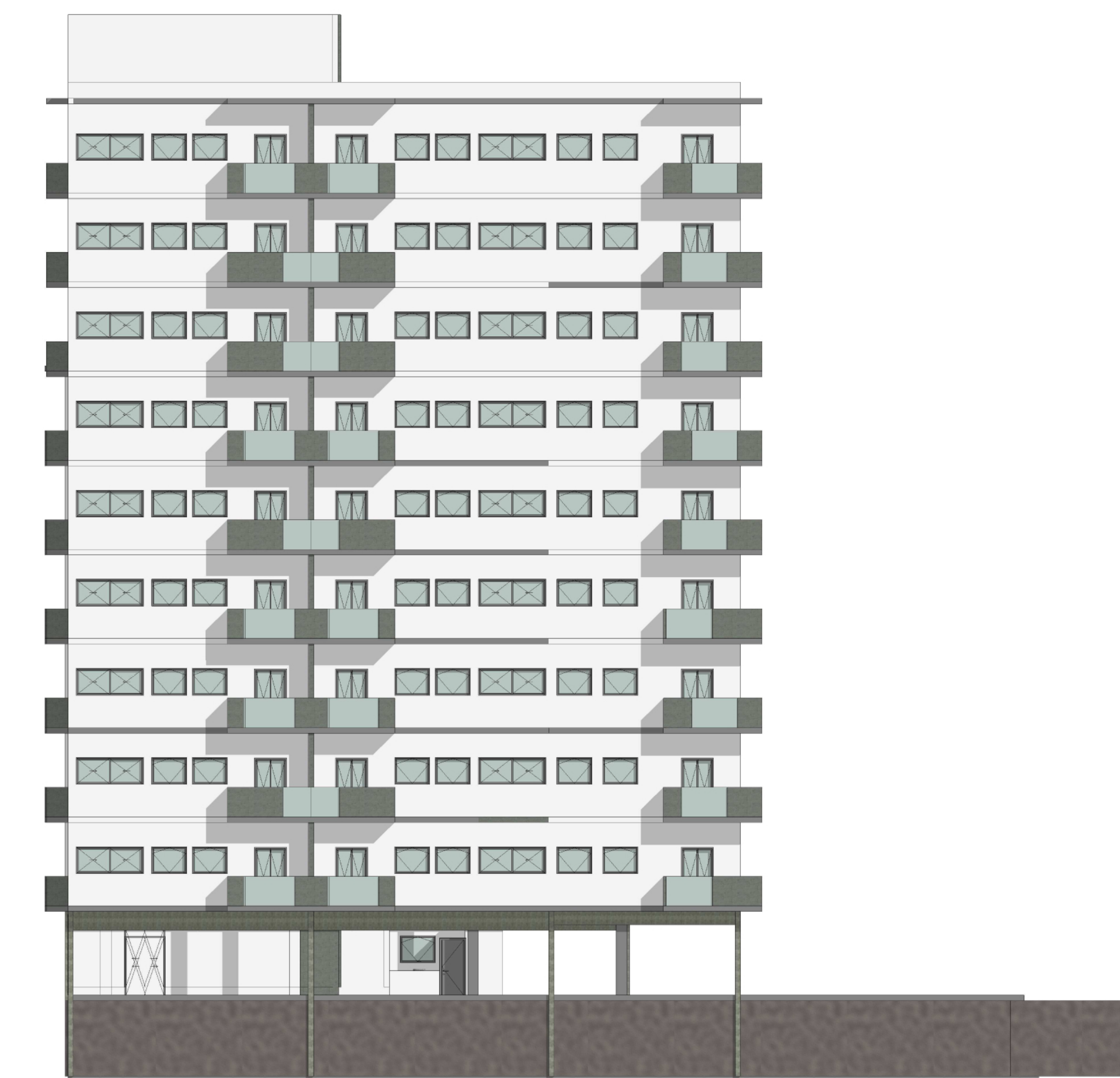
Elevação Leste esc: 1:125
