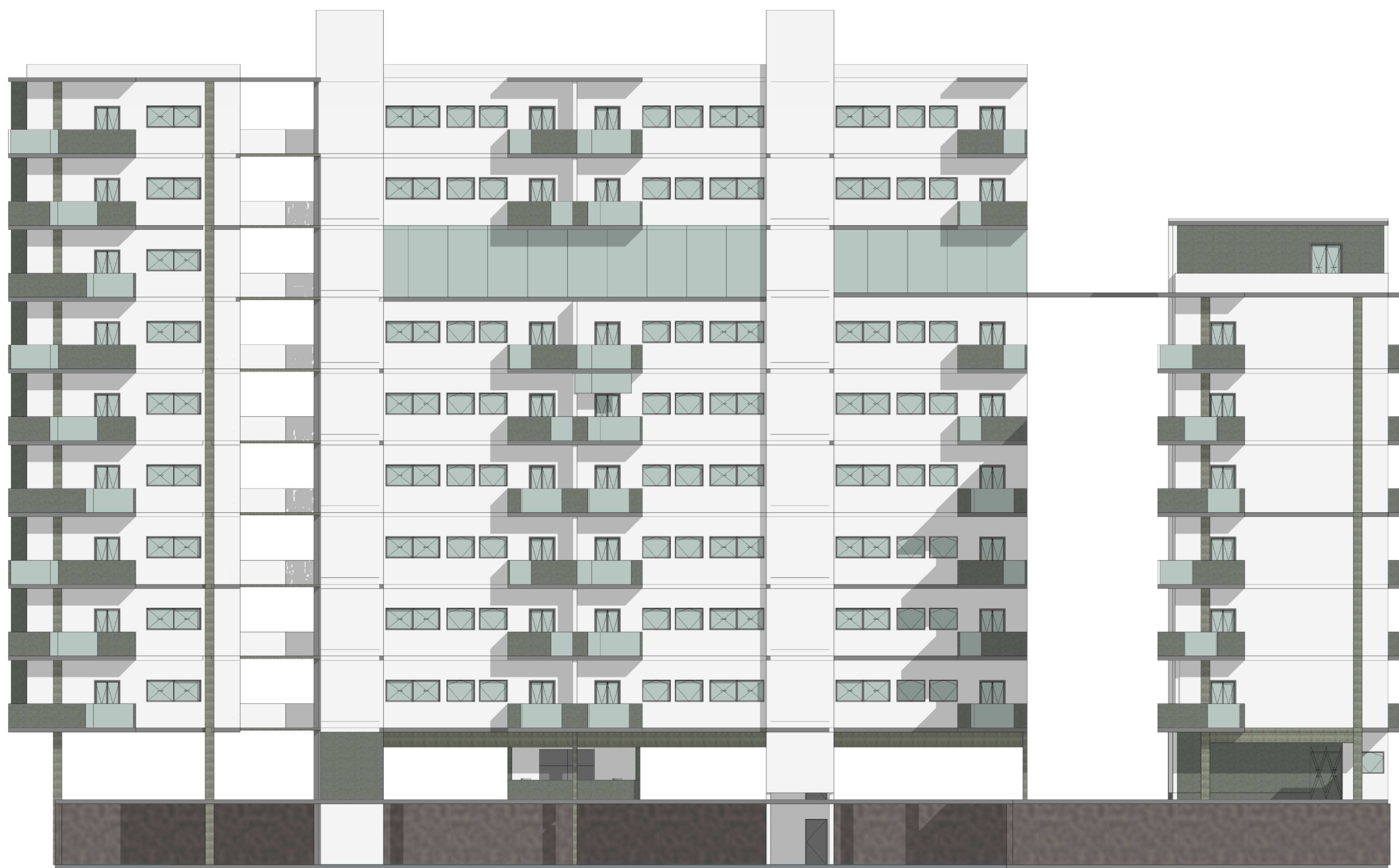
Elevação Sul esc: 1:125
